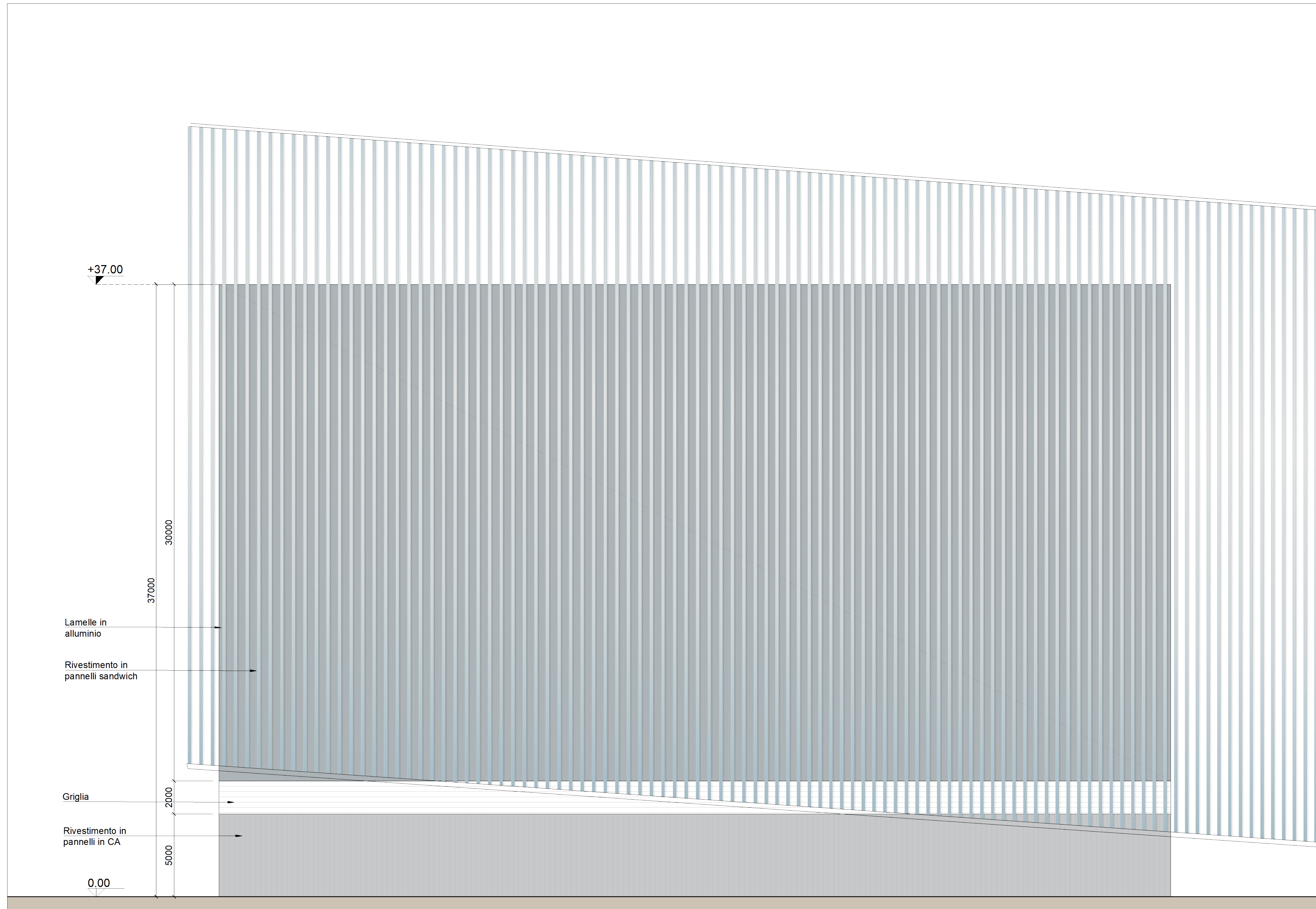
Prospetto P-01 Scala 1:100
