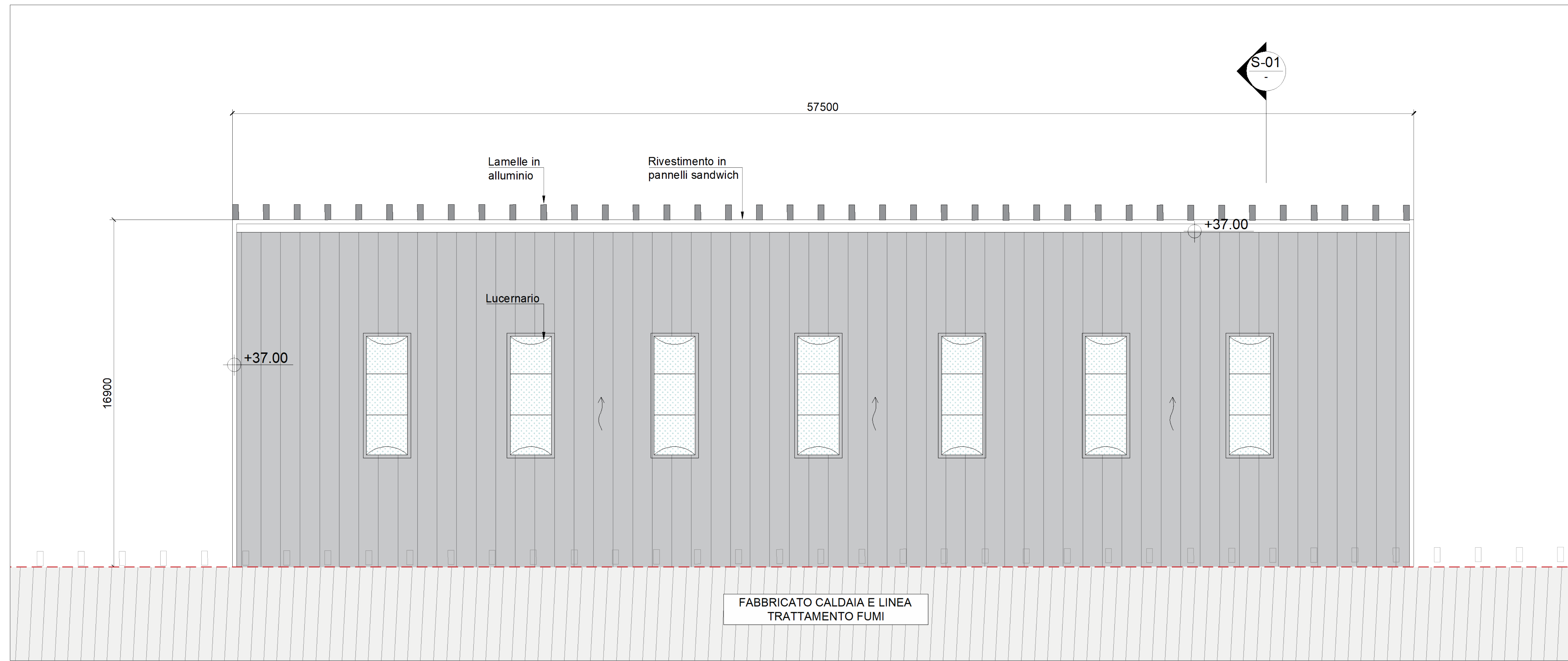
Pianta copertura Scala 1:100
