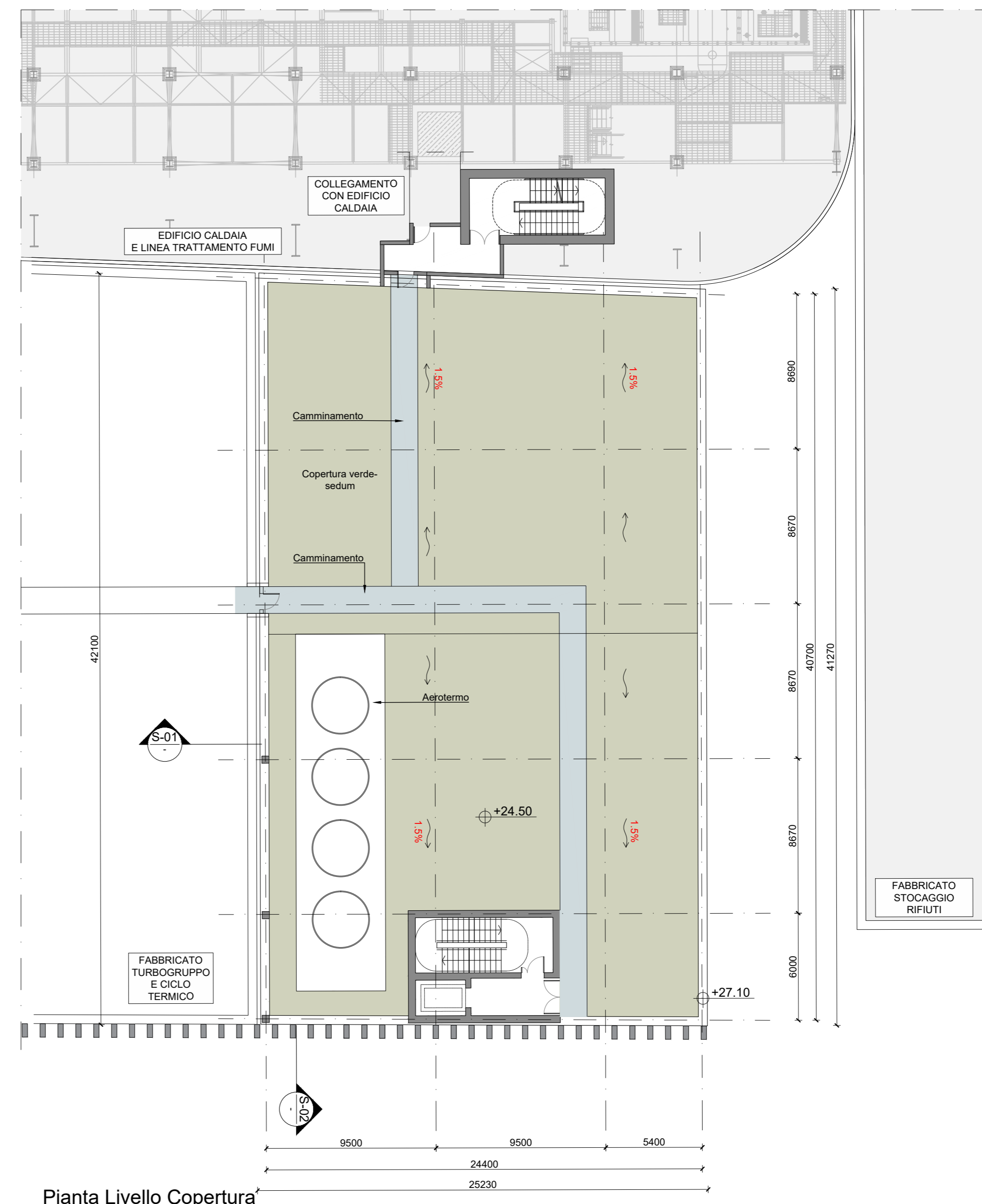
Pianta Livello Copertura Scala 1:200
