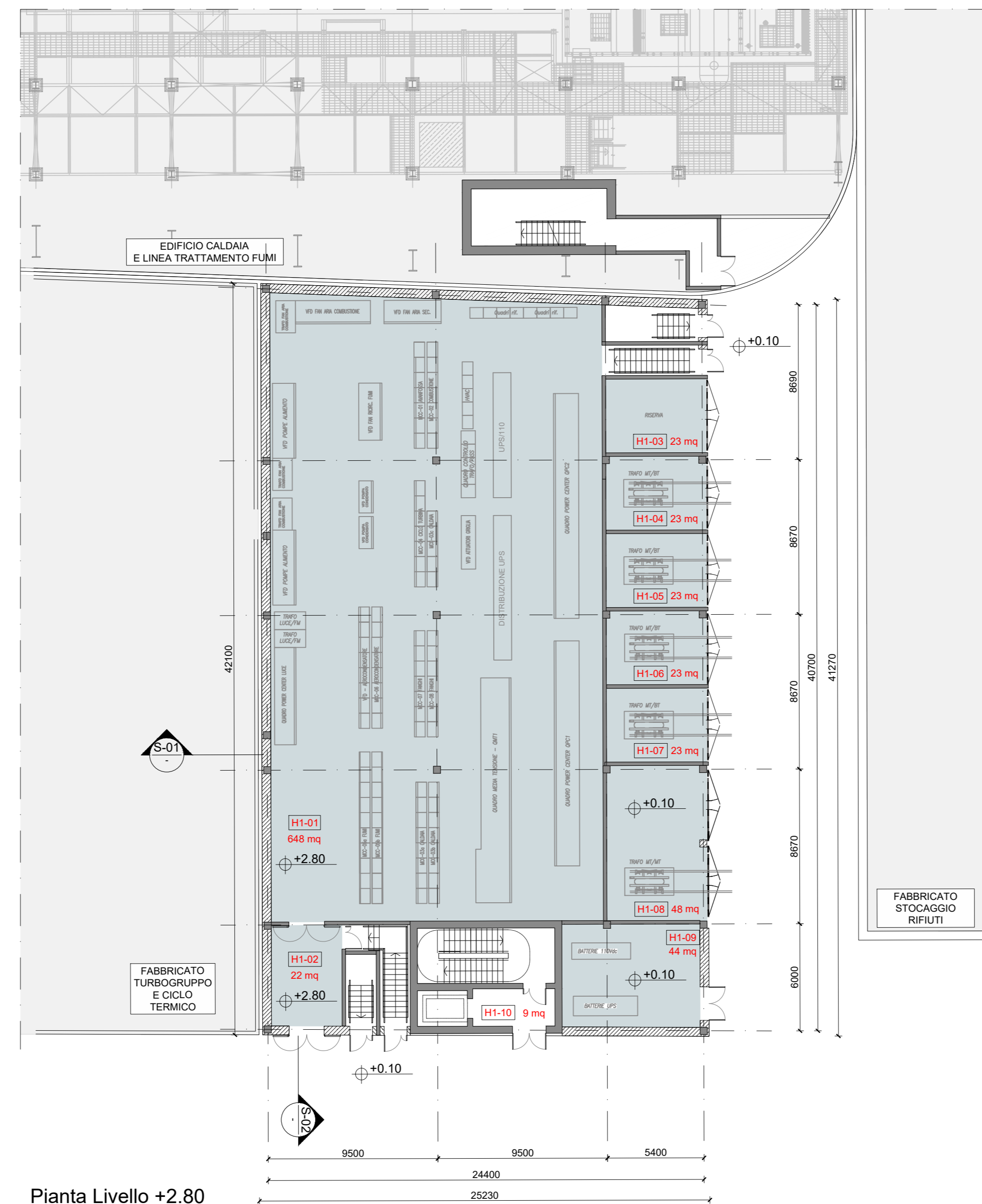
Pianta Livello +2.80 Scala 1:200
