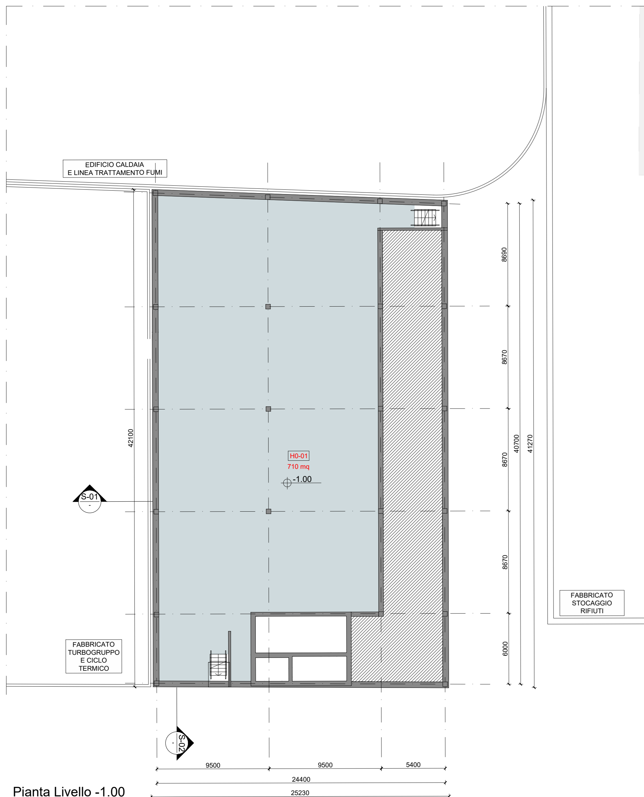
Pianta Livello -1.00 Scala 1:200
