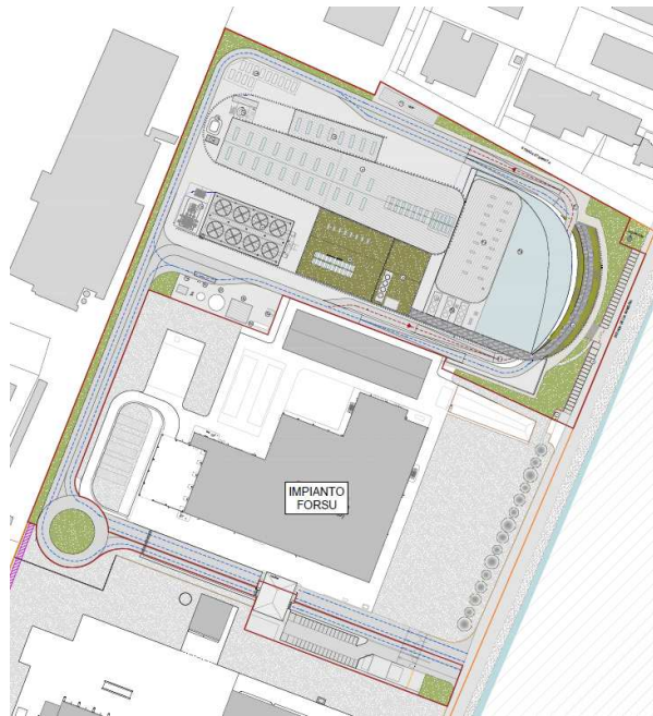
Figura 4 planimetria generale di progetto
