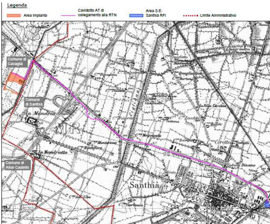
Figura 2 Percorso elettrodotto
