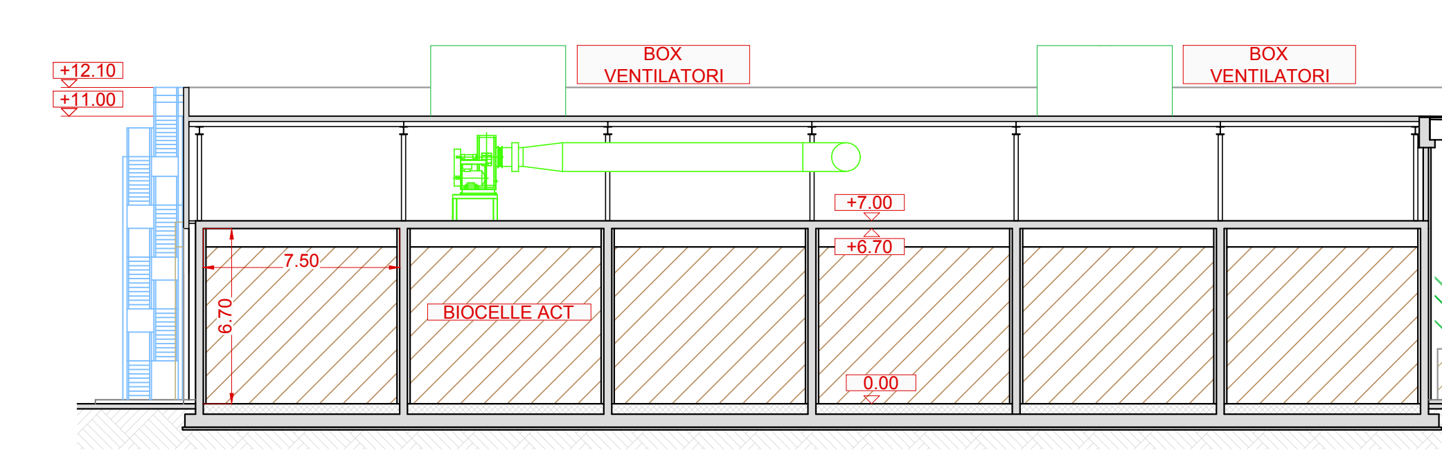
SEZIONE B-B
