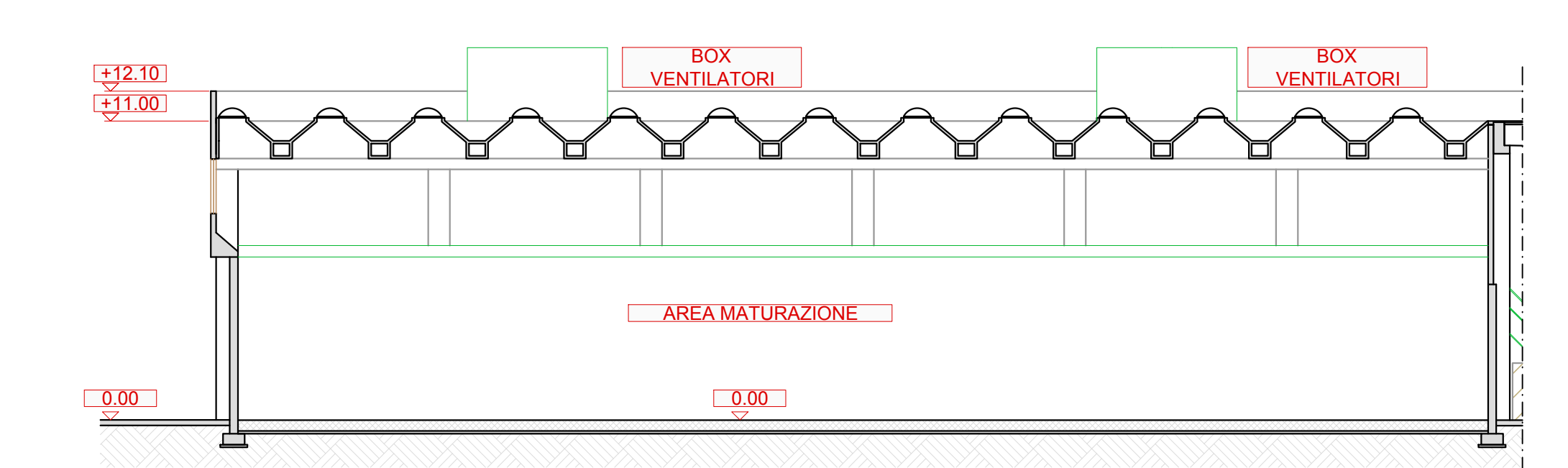
SEZIONE C-C
