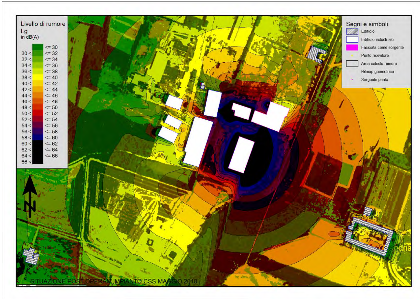
Figura 1 Situazione ANTE OPERAM IMPIANTO CSS e PLASTICHE
