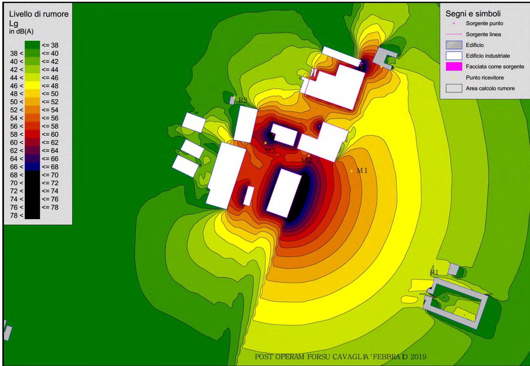
Figura 2 Post operam impianto FORSU
