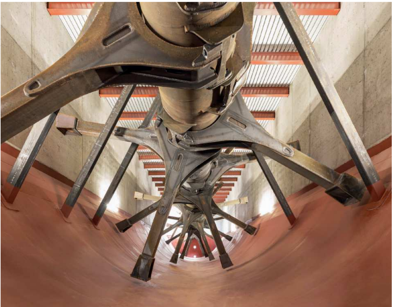
Esempio di digestore con albero longitudinale e pale
