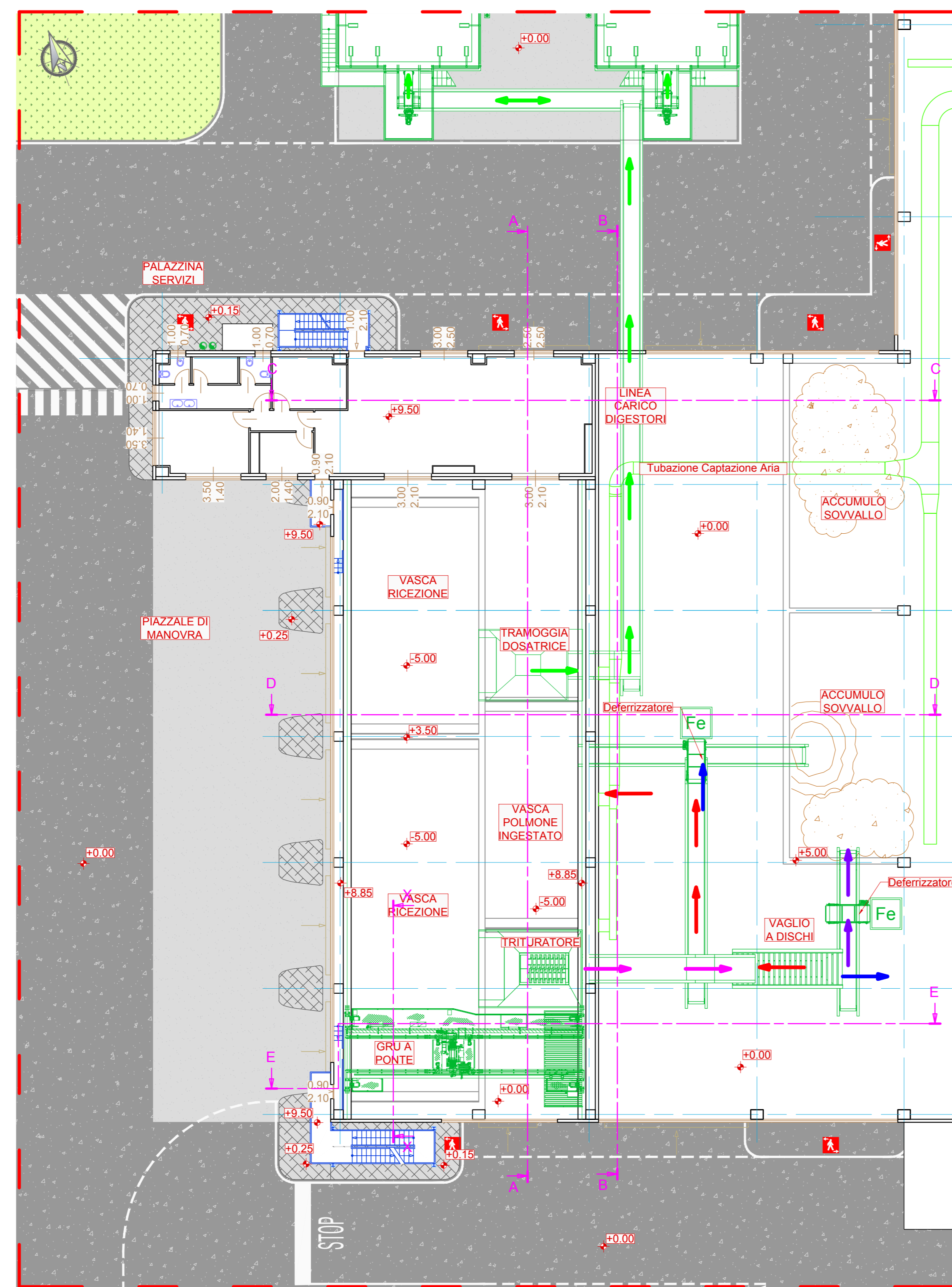
PIANTA VIE DI CORSA +9.50
