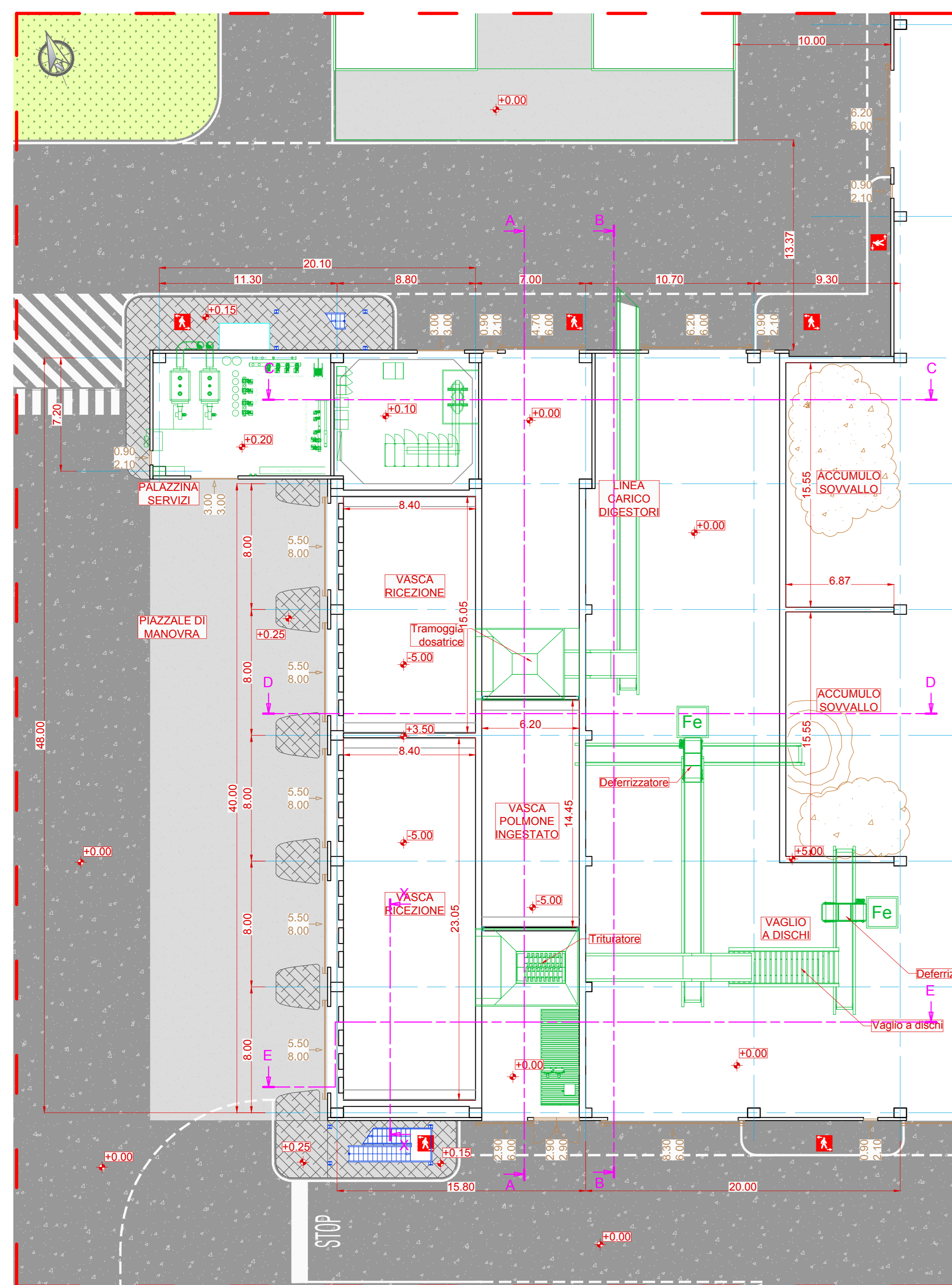
PIANTA PIANO TERRA
