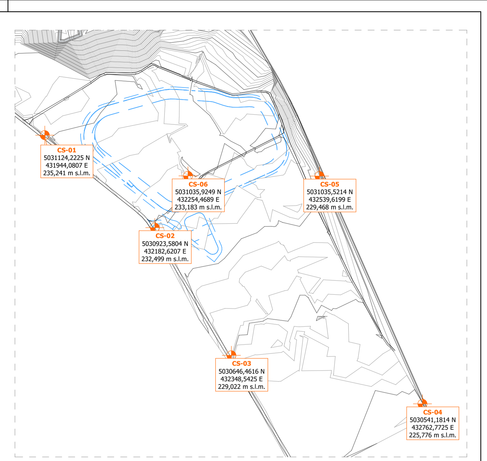
Planimetria capisaldi 1:5000
