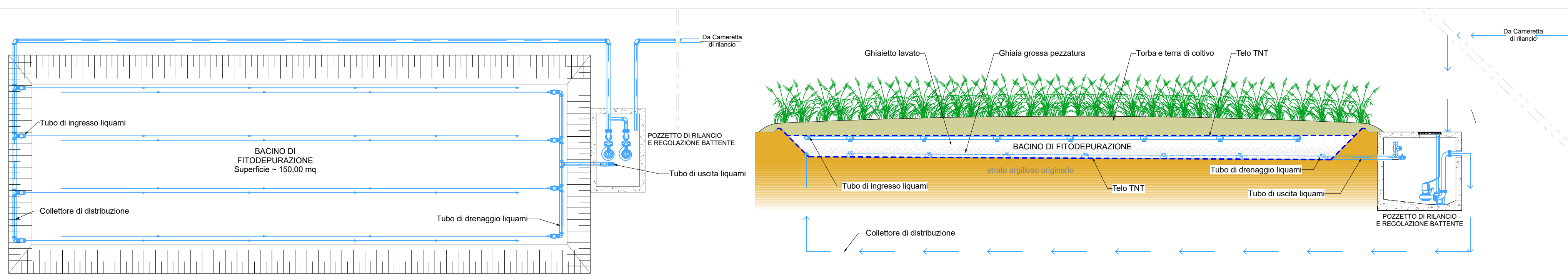
DETTAGLIO SISTEMA DI FITODEPURAZIONE scala 1:100
